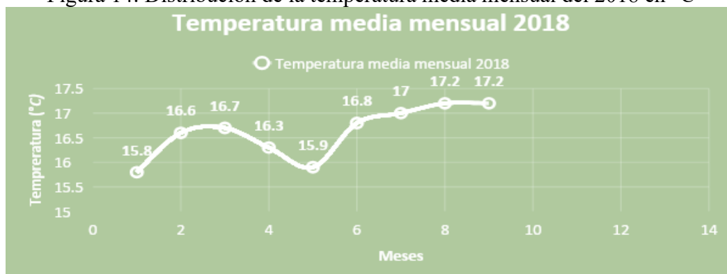
Figura 14: Distribución de la temperatura media mensual del 2018 en °C
