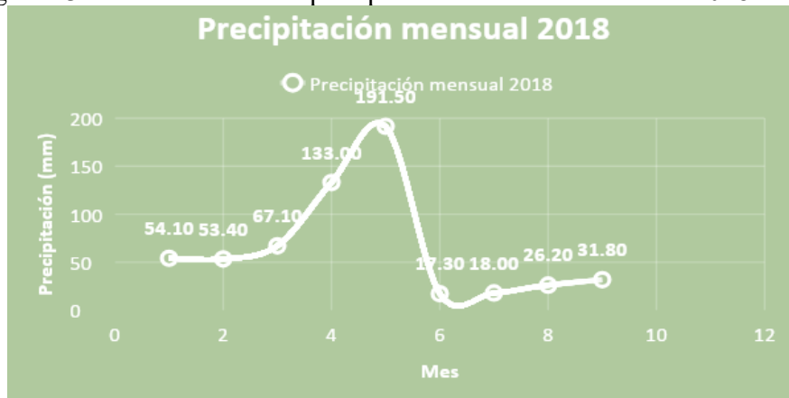
Figura 13: Distribución de la precipitación mensual durante el 2018 en mm
