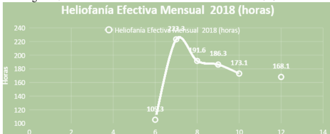
Figura 17: Distribución de heliofanía efectiva mensual del 2018 en horas
